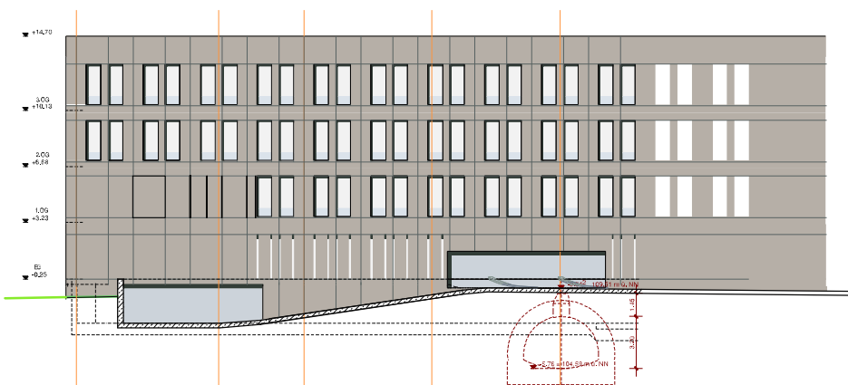
HMDF, Wiesbaden 2014 Original-Bemusterung der Kombinationslösung mCon-UK + ACT Fischer Hinterschnitt-Technik
