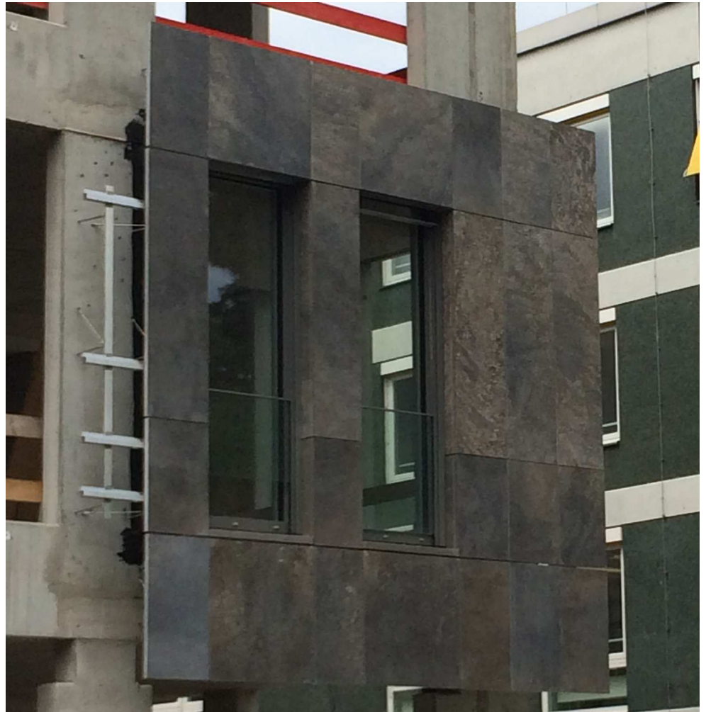
HMDF, Wiesbaden 2014 Original-Bemusterung der Kombinationslösung mCon-UK + ACT Fischer Hinterschnitt-Technik
